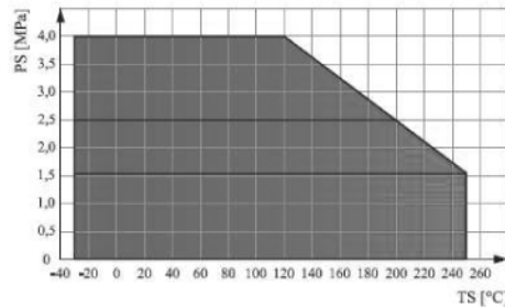
Wykres pola pracy kurka / Pressure-temperature limits / Связь между температурой и давлением
